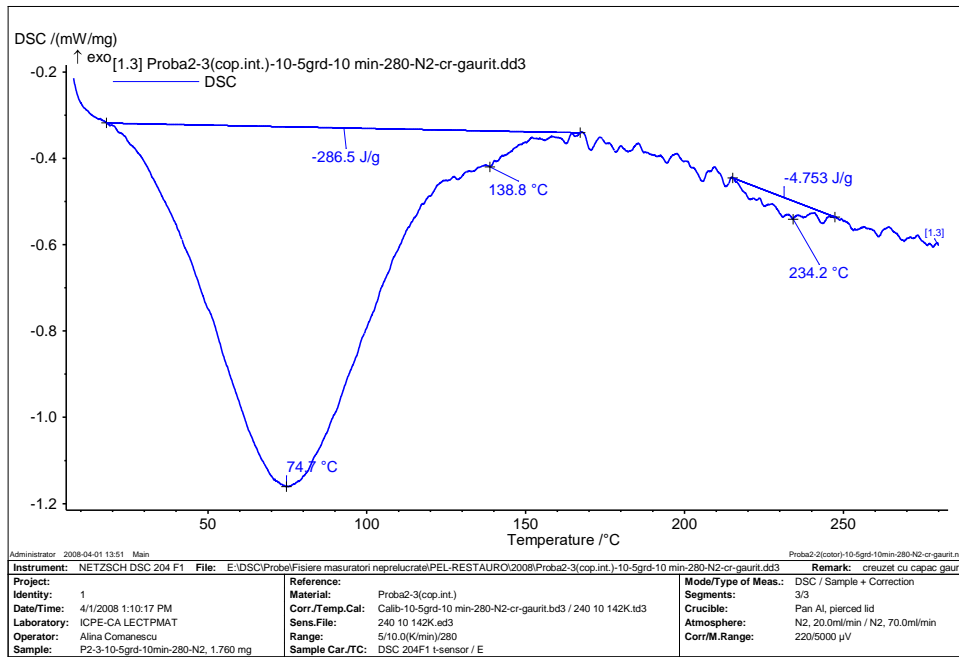
Fig. 1.6. Curba DSC pentru proba de piele P2-3
