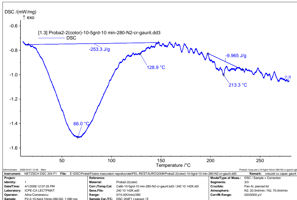
Fig. 1.5. Curba DSC pentru proba de piele P2-2
