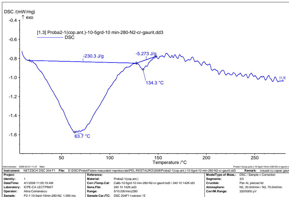
Fig. 1.4. Curba DSC pentru proba de piele P2-1
